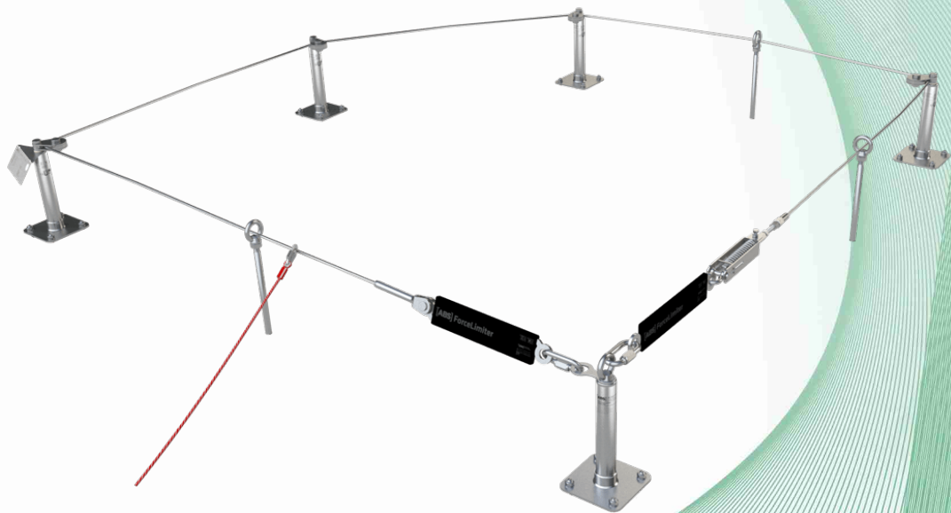
Bild 1: Anschlagereinrichtung, Typ: ABS-Lock® SYS I, Montagebeispiel für nicht überfahrbares Drahtseilsystem mit Führung Ø 8 mm
