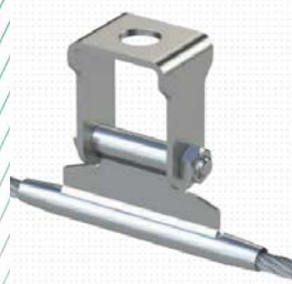
Bild 14: Zwischenhalter - S für Überkopfanwendung für Führung Ø 8 mm
